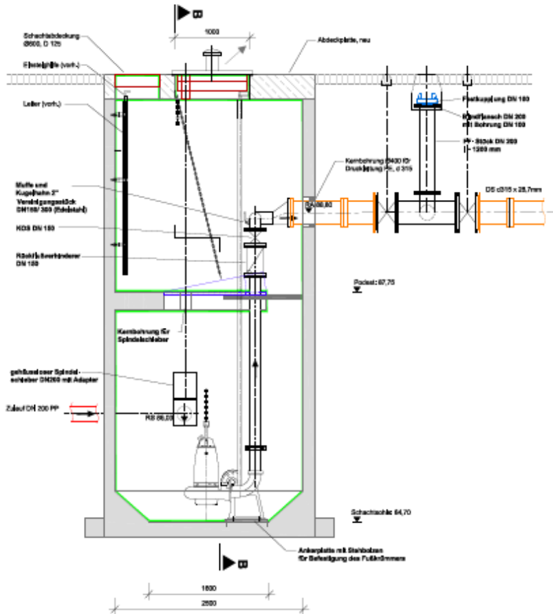
Schnitt A-A
