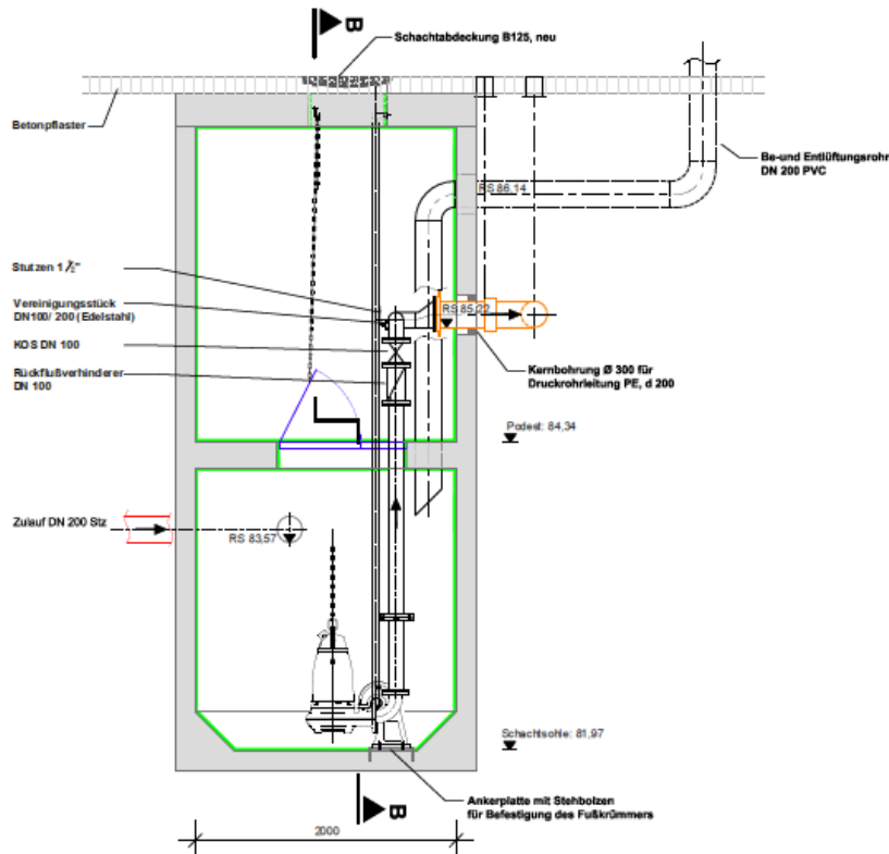
Schnitt A - A
