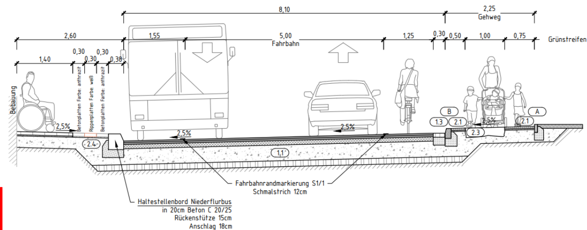
Regelquerschnitt 2-2
